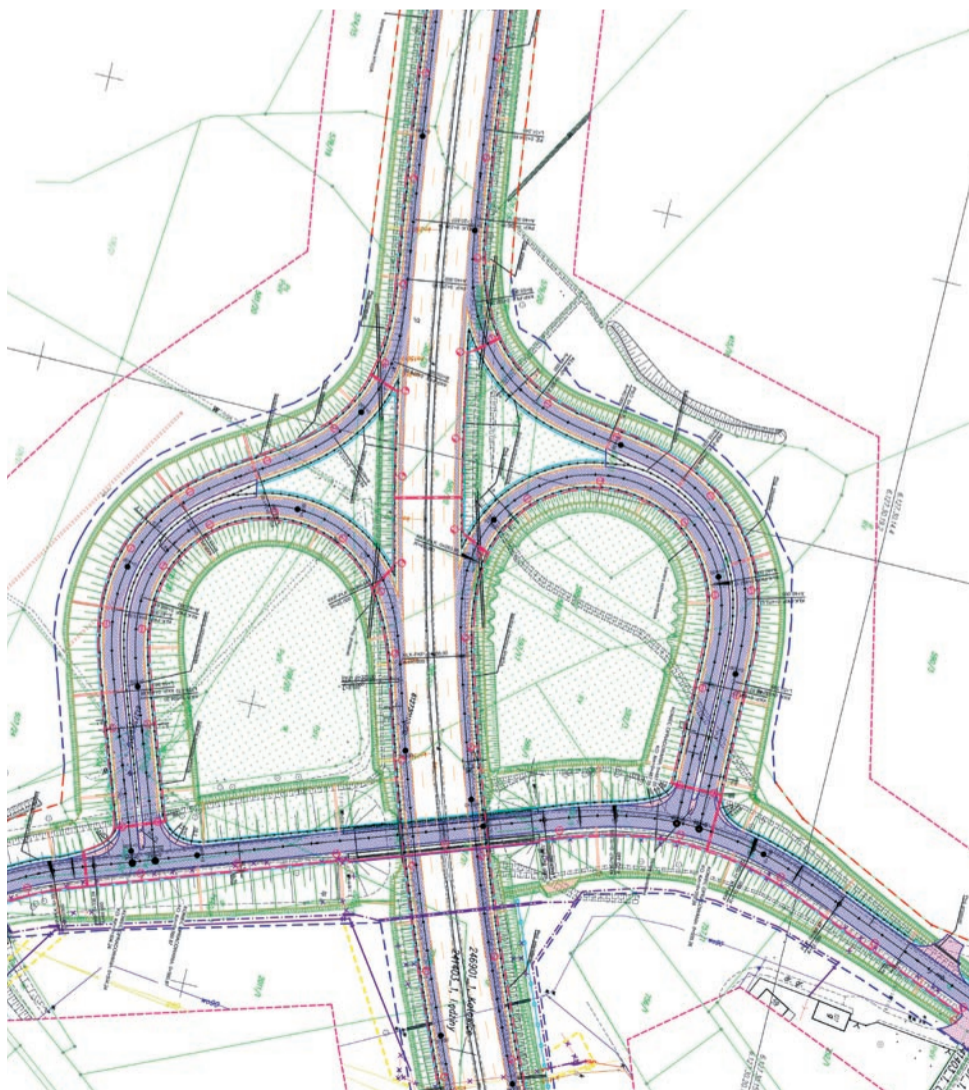
Projekt węzła drogowego „Olszyce”
